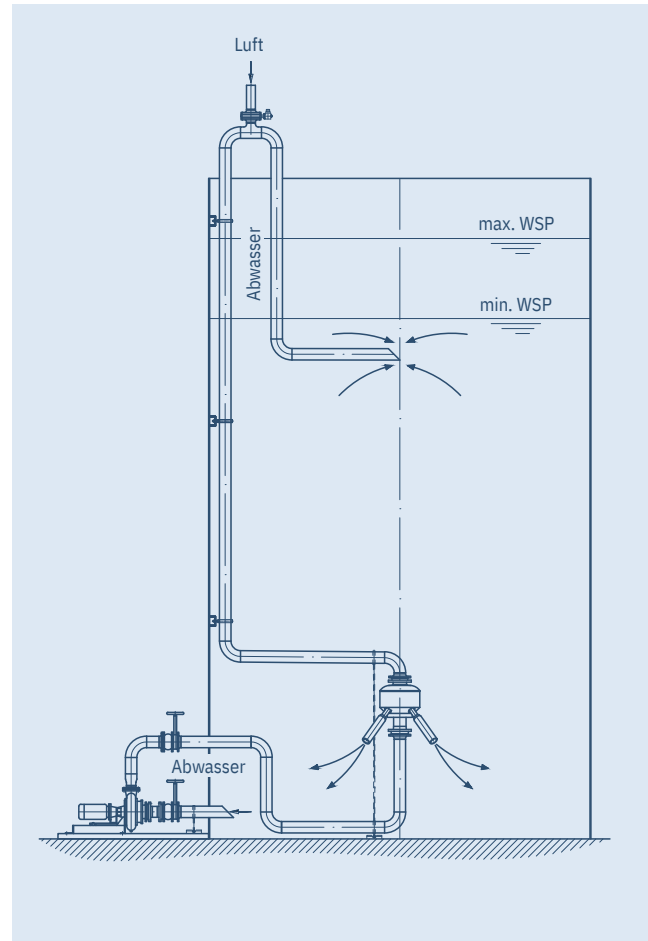
SBR mit atmosphärischer Luftansaugung
