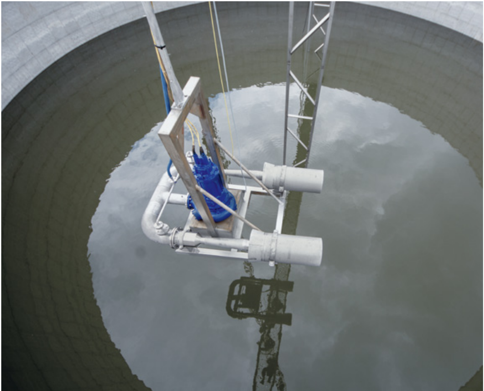
Mobiles Sauerstoffeintragungssystem beim Absenken in die Kläranlage eines Obst und Gemüse verarbeitenden Betriebs in Belgien. Der Einbau erfolgte bei laufendem Anlagenbetrieb durch die Westfalen AG. (Bilder © Westfalen AG, www.westfalen.com )
