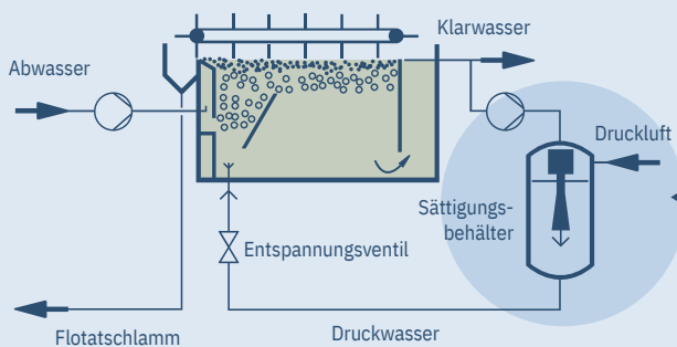
Druckentspannungsflotation als Nachklärung in einer biologischen Abwasserreinigungsanlage
