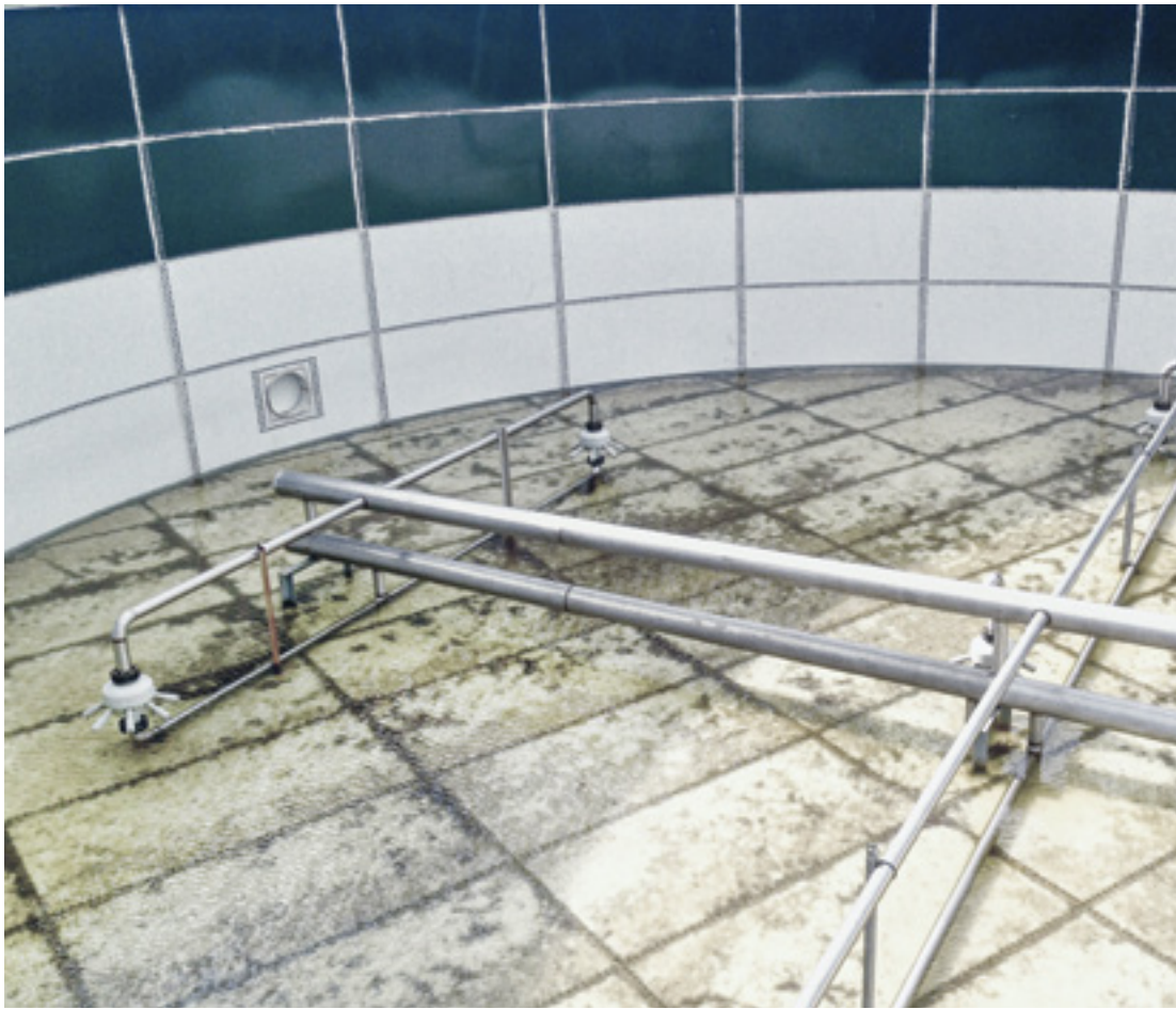
Siebenstrahlige Ejektoren in einem 2.200 m 3 Belebungsbecken in der Speiseölindustrie in Brasilien
